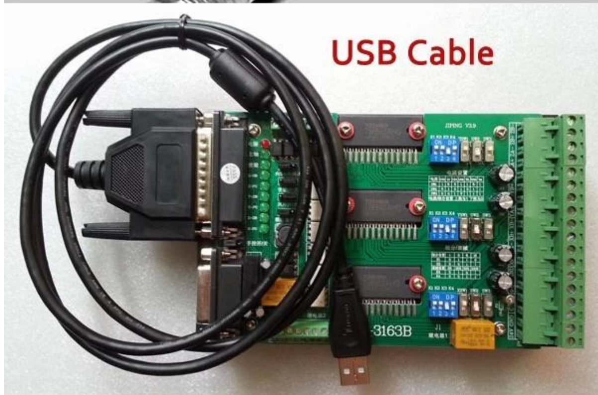
CNC 6090 Mini ЧПУ гравировальный станок 3 Ось
