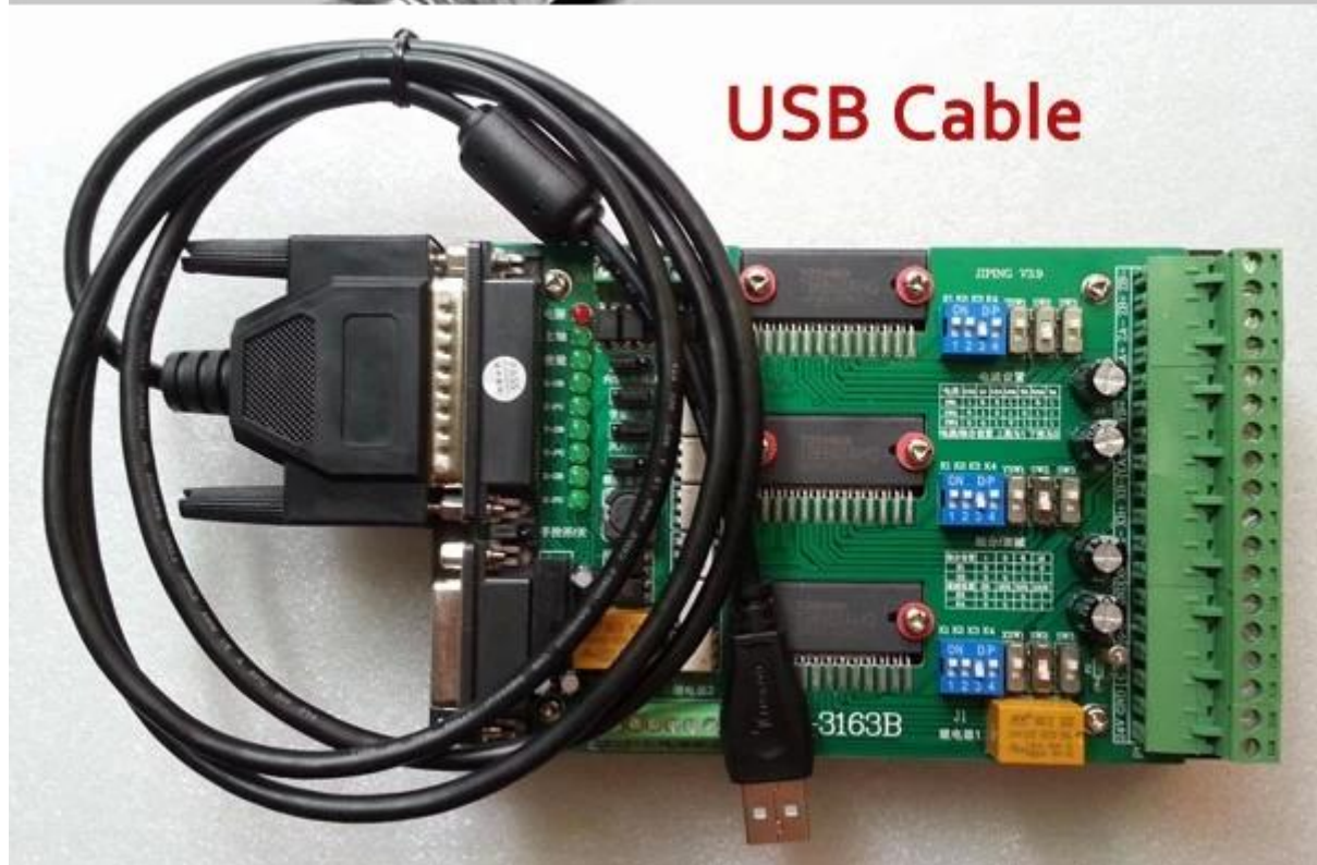
CNC 6090 Mini CNC Engraving Machine 3 Axis
